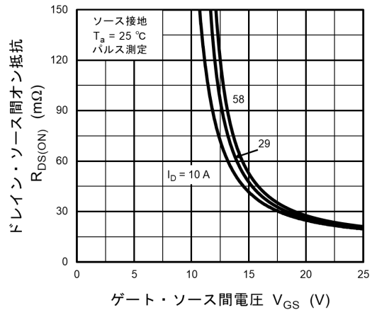
図 8.8 R_{DS(ON)} - V_{GS}
