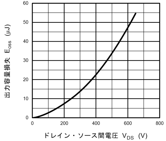
図 8.14 E_{oss} - V_{DS}
