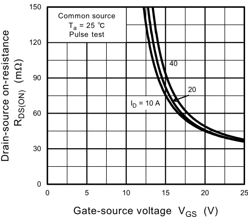
Fig. 8.8 R_{DS(ON)} - V_{GS}
