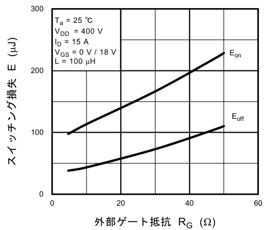
図 8.16 E - R_G
