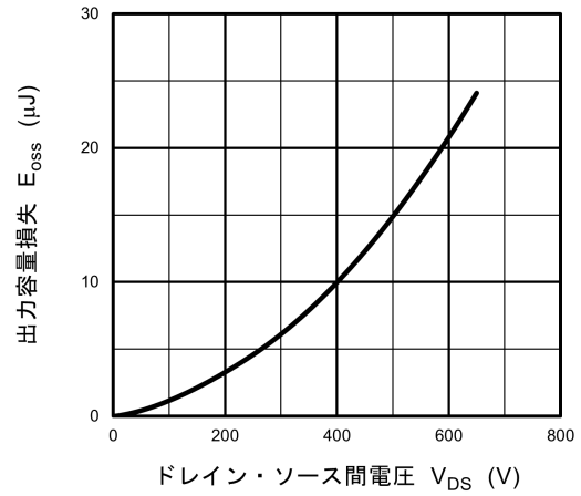
図 8.14 E_{oss} - V_{DS}
