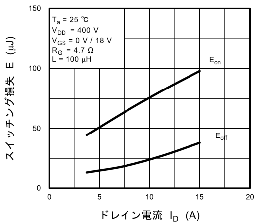
図 8.15 E - I_D
