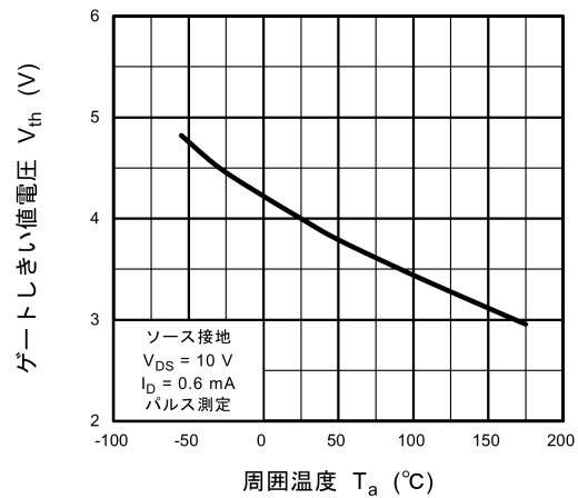
図 8.4 V_{th} - T_a
