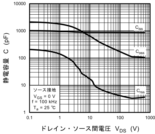
図 8.13 C - V_{DS}
