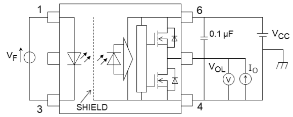
図 13.1.3 V_{OL} 測定回路
