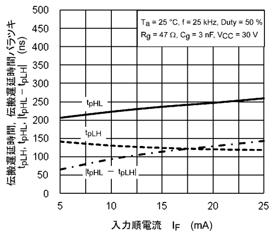
図 13.2.13 t_{pLH}, t_{pHL}, |t_{pHL} - t_{pLH}| - I_F
