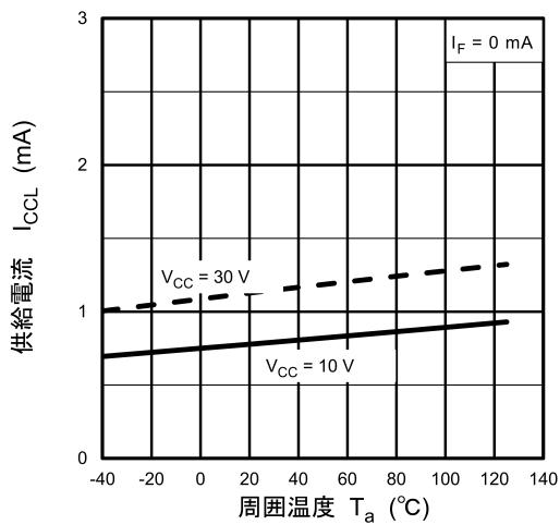
図 13.2.5 I_{CCL} - T_a
