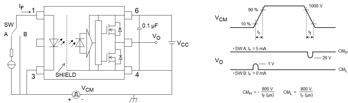
図 13.1.7 コモンモード過渡耐性測定回路, 波形
