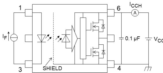
図 13.1.4 I_{CCH} 測定回路
