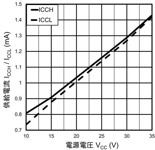
図 13.2.7 I_{CC} - V_{CC}
