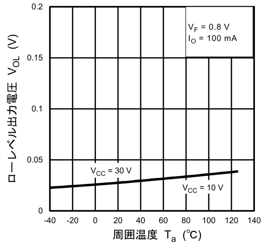
図 13.2.8 V_{OL} - T_a
