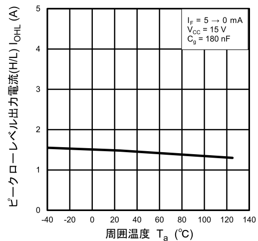
図 13.2.10 I_{OHL} - T_a
