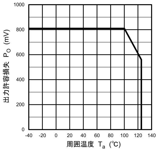
図 13.2.3 P_O - T_a
