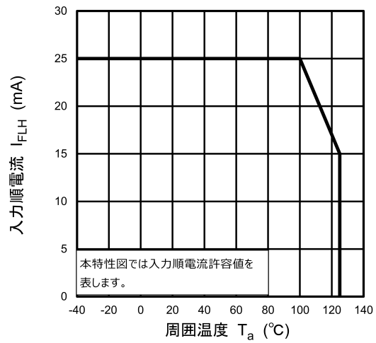
図 13.2.2 I_F - T_a
