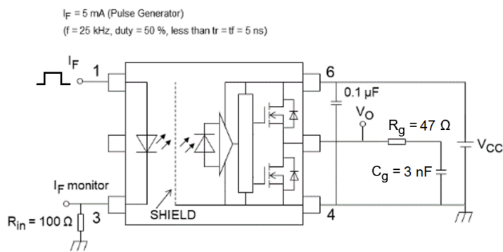
図 13.1.6 伝搬遅延時間測定回路, 波形
