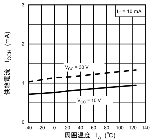
図 13.2.6 I_{CCH} - T_a
