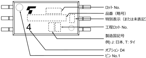
図 17.4 現品表示例 (注)
