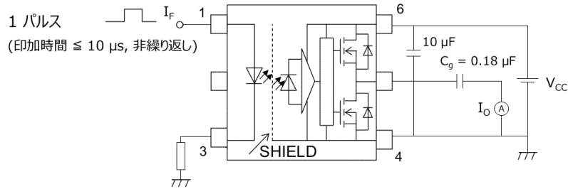
図 13.1.1 I_{OLH} , I_{OLH} 測定回路
