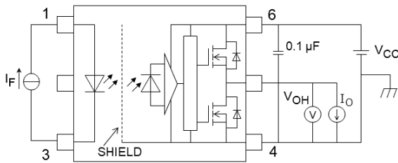
図 13.1.2 V_{OH} 測定回路
