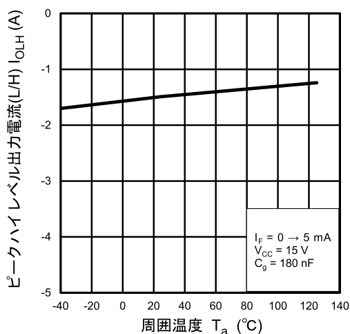
図 13.2.11 I_{OLH} - T_a
