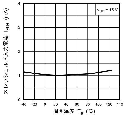
図 13.2.4 I_{FLH} - T_a
