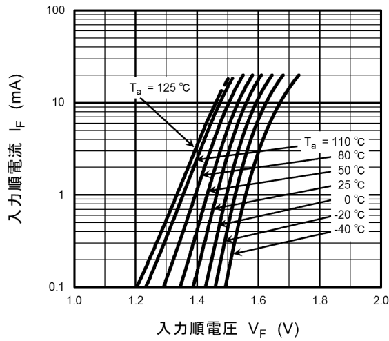
図 13.2.1 I_F - V_F
