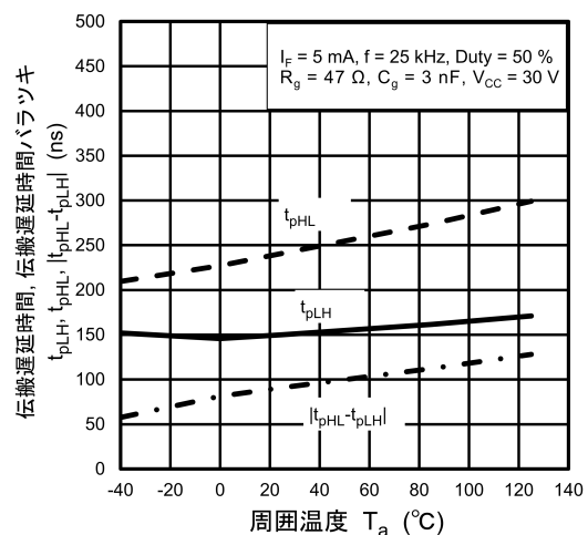
図 13.2.12 t_{pLH}, t_{pHL}, |t_{pHL} - t_{pLH}| - T_a
