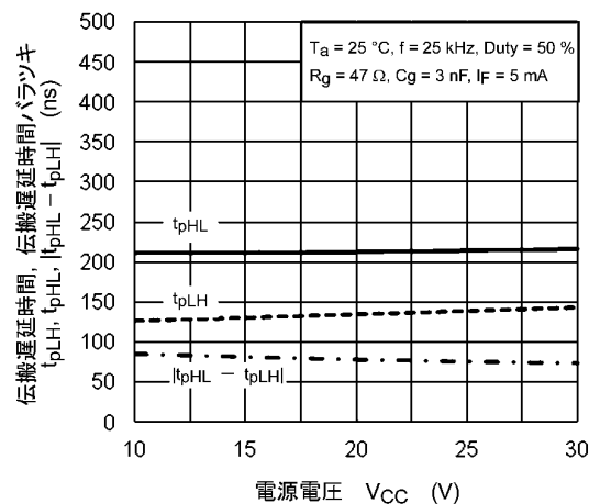
図 13.2.14 t_{pLH}, t_{pHL}, |t_{pHL} - t_{pLH}| - V_{CC}
