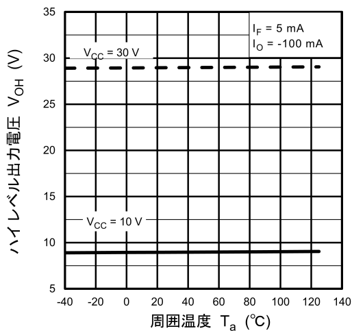
図 13.2.9 V_{OH} - T_a
