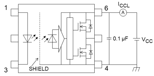
図 13.1.5 I_{CCL} 測定回路
