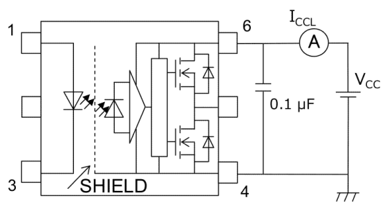
図 13.1.5 ICCL測定回路
