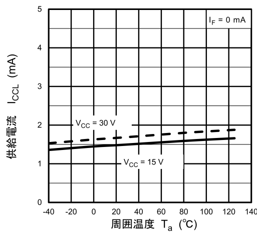
図 13.2.5 I_{CCL} - T_a
