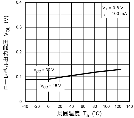
図 13.2.8 V_{OL} - T_a
