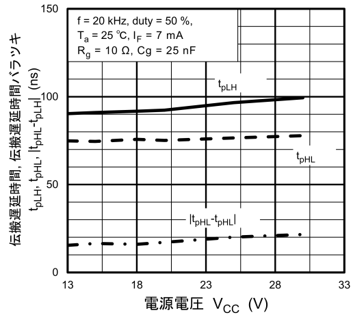
図 13.2.14 t_{pLH} , t_{pHL} , |t_{pHL} - t_{pLH}| - V_{CC}
