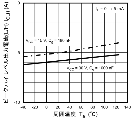
図 13.2.10 I_{OLH} - T_a
