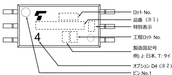
図 17.3 現品表示例
