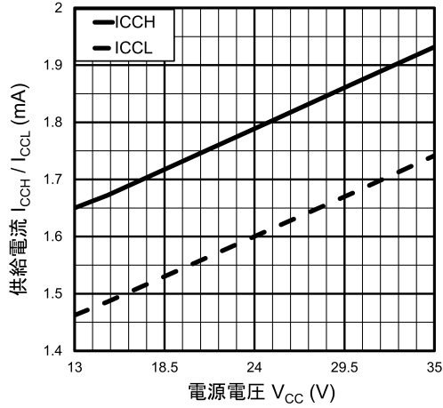
図 13.2.7 I_{CC} - V_{CC}
