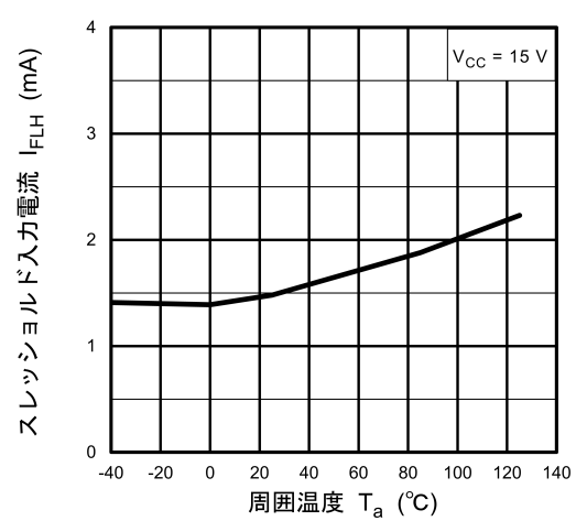
図 13.2.4 I_{FLH} - T_a
