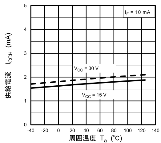
図 13.2.6 I_{CCH} - T_a
