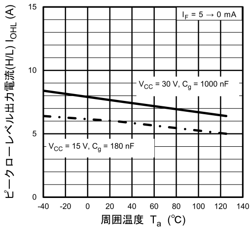
図 13.2.11 I_{OHL} - T_a
