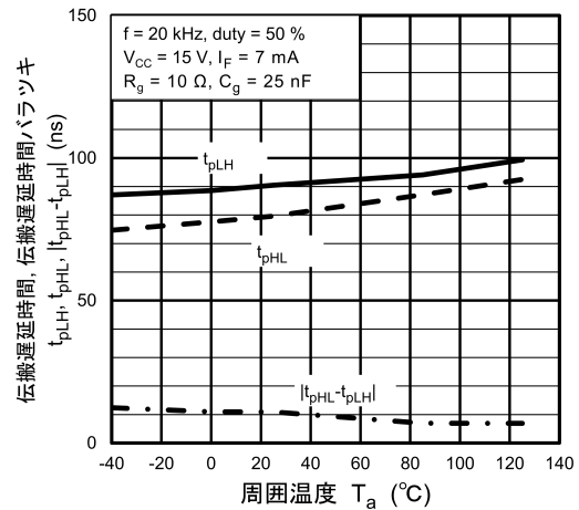
図 13.2.12 t_{pLH} , t_{pHL} , |t_{pHL} - t_{pLH}| - T_a
