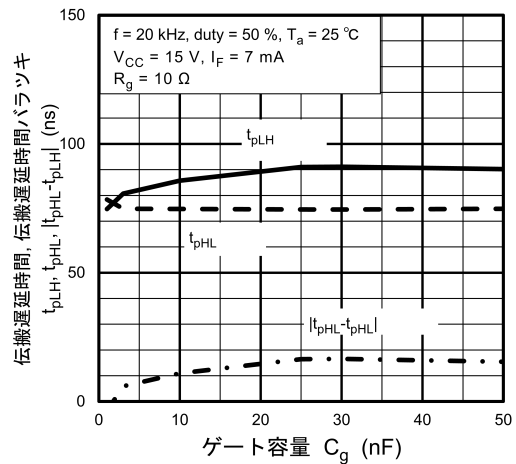
図 13.2.16 t_{pLH} , t_{pHL} , |t_{pHL} - t_{pLH}| - C_g
