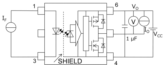
図 13.1.2 V OH 測定回路
