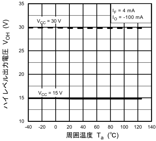
図 13.2.9 V_{OH} - T_a
