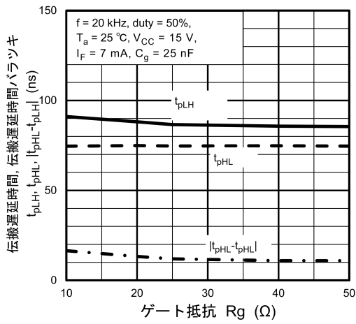
図 13.2.15 t_{pLH} , t_{pHL} , |t_{pHL} - t_{pLH}| - R_g
