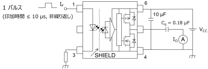
図 13.1.1 I OLH , I OH 測定回路
