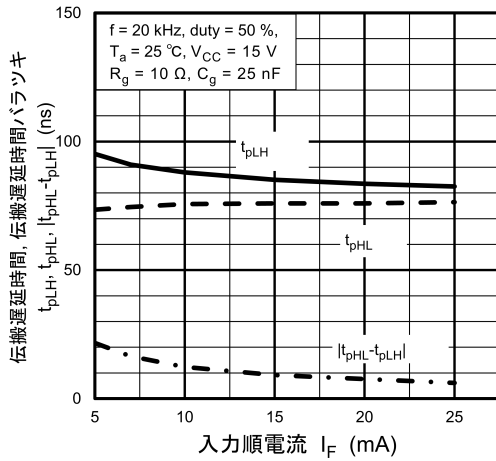
図 13.2.13 t_{pLH} , t_{pHL} , |t_{pHL} - t_{pLH}| - I_F
