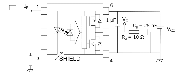
図 13.1.6 伝搬遅延時間測定回路, 波形
