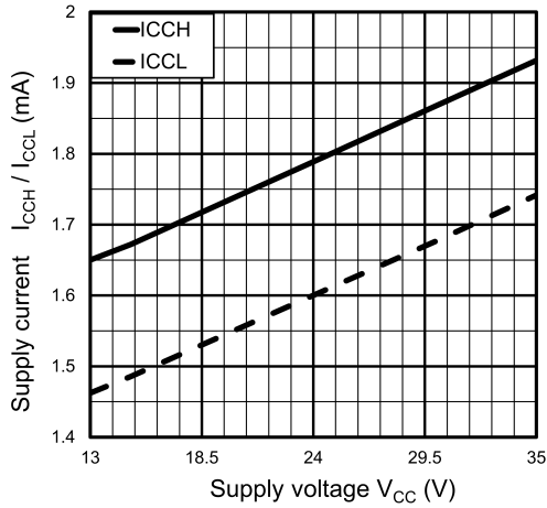
Fig. 13.2.7 I_{CC} - V_{CC}
