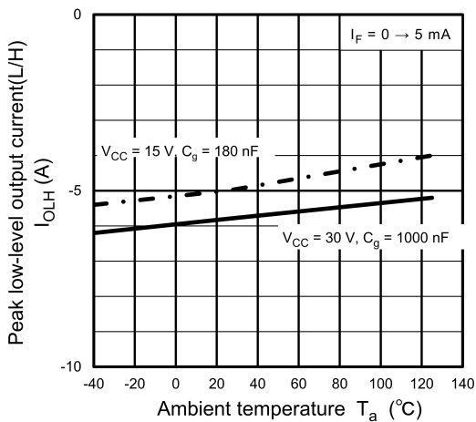
Fig. 13.2.11 I_{OHL} - T_a
