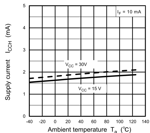
Fig. 13.2.6 I_{CCH} - T_a
