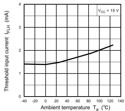
Fig. 13.2.4 I_{FLH} - T_a
