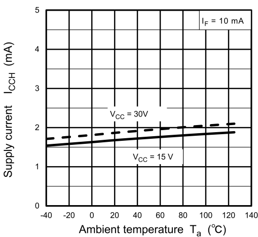
Fig. 13.2.6 I_{CCH} - T_a
