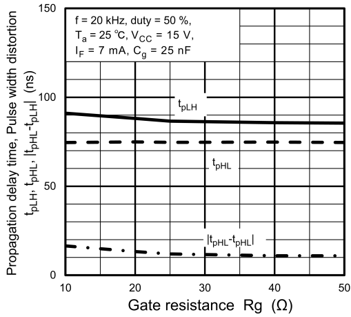
Fig. 13.2.15 t_{pLH} , t_{pHL} , |t_{pHL}-t_{pLH}| - R_g
