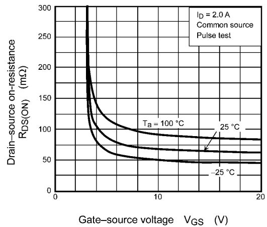
Fig. 9.4 R_{DS(ON)} - V_{GS}
