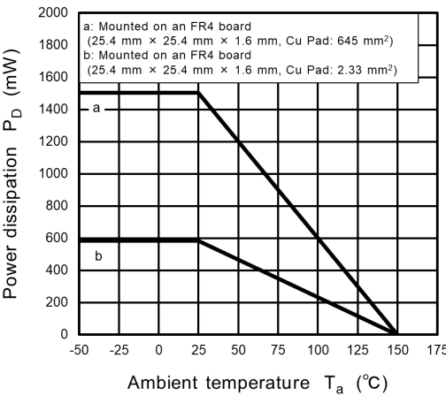
Fig. 7.10 P_D - T_a
