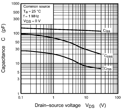
Fig. 7.8 C - V_{DS}
