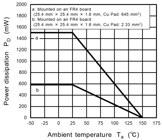
Fig. 9.10 P_D - T_a
