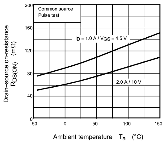
Fig. 9.6 R_{DS(ON)} - T_a
