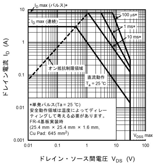
図 9.11 安全動作領域
