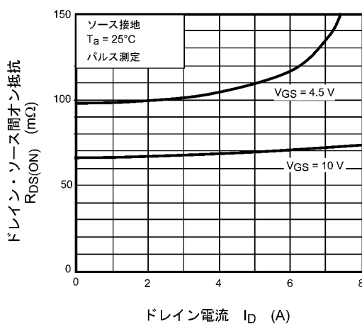
図 9.5 R_{DS(ON)} - I_D
