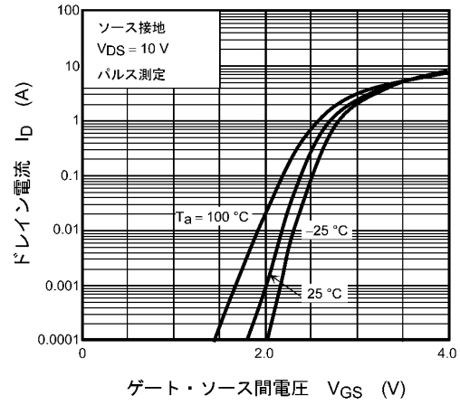
図 9.2 I_D - V_{GS}
