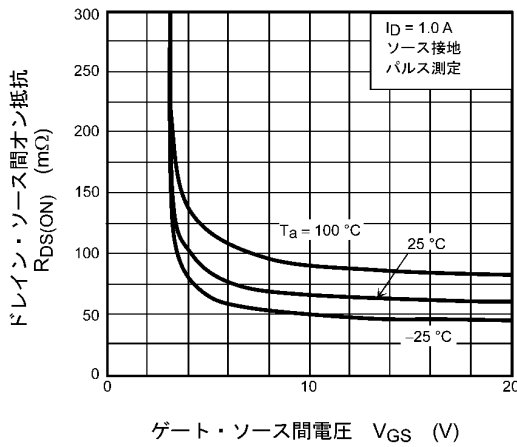
図 9.3 R_{DS(ON)} - V_{GS}
