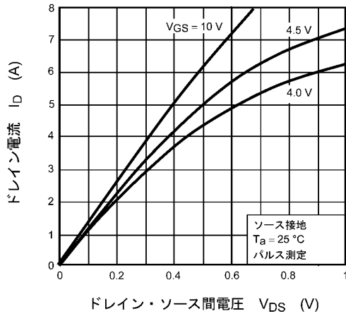
図 9.1 I_D - V_{DS}
