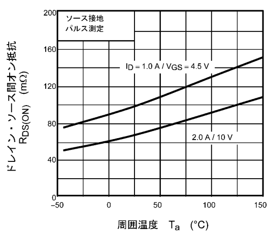
図 9.6 R_{DS(ON)} - T_a
