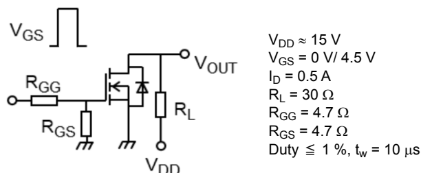
図 6.2.1 スイッチング時間の測定回路
