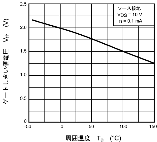
図 9.7 V_{th} - T_a
