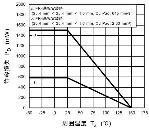
図 9.10 P_D - T_a
