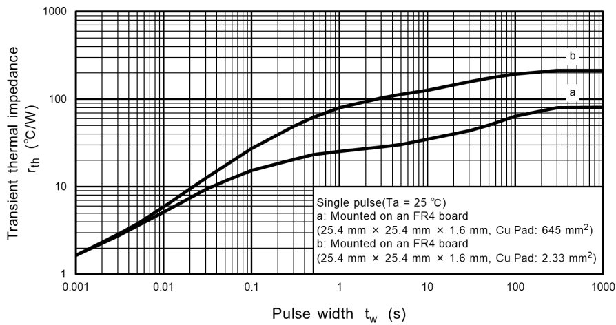
Fig. 9.9 r_{th} - t_w
