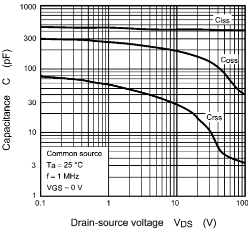
Fig. 9.7 C - V_{DS}
