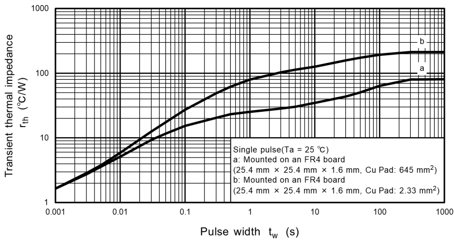
Fig. 9.9 r_{th} - t_w
