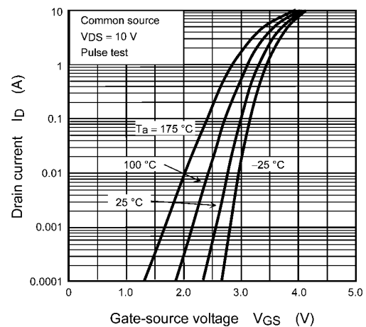
Fig. 7.2 ID - VGS
