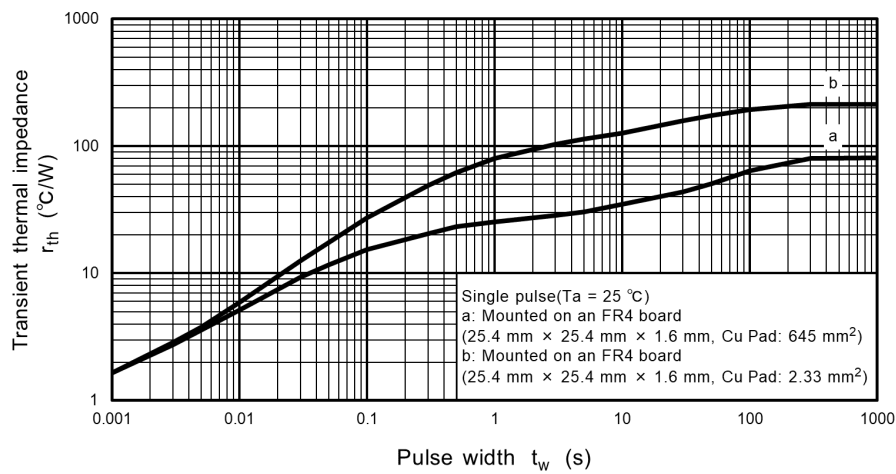
Fig. 7.9 r_{th} - t_w
