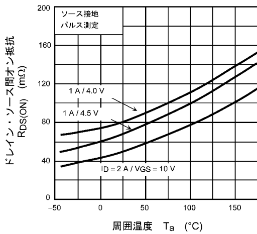
図 9.5 R_{DS(ON)} - T_a
