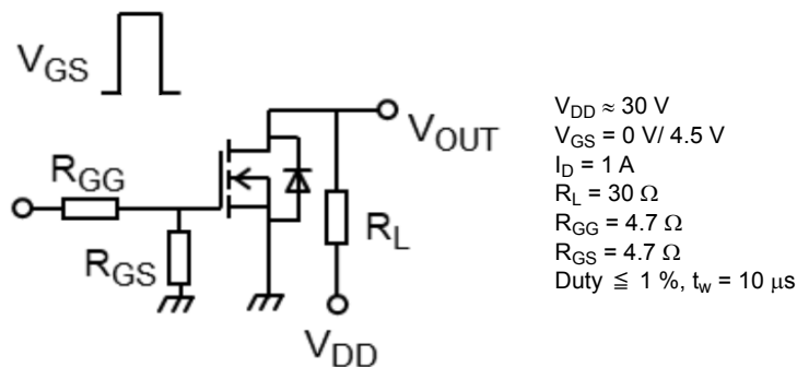
図 6.2.1 スイッチング時間の測定回路
