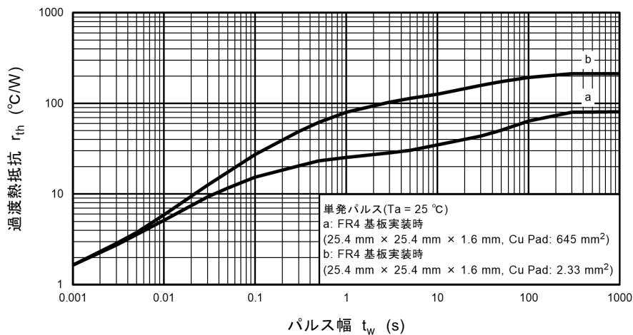
図 9.11 r th - t w
