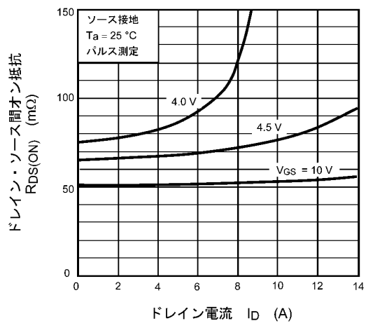
図 9.4 R_{DS(ON)} - I_D
