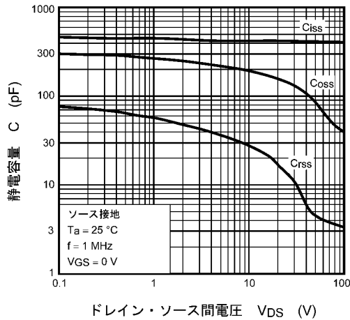
図 9.7 C - V DS
