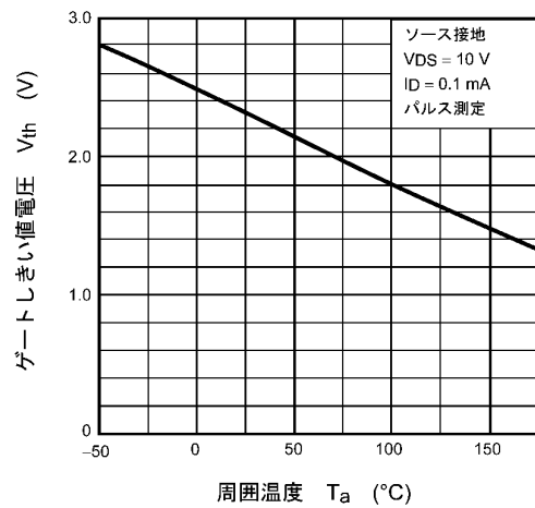
図 9.6 V_{th} - T_a
