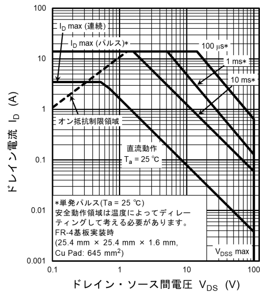
図 9.10 安全動作領域
