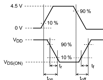
図 6.2.2 入力波形/出力波形
