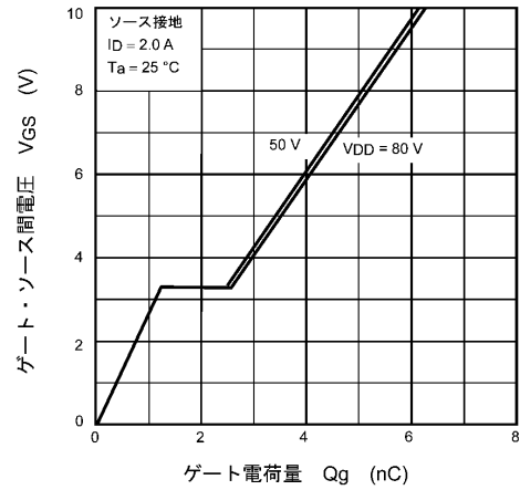
図 9.8 ダイナミック入力特性
