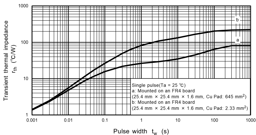
Fig. 9.11 r_{th} - t_w
