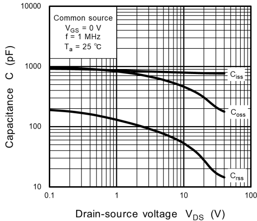
Fig. 9.7 C - V_{DS}
