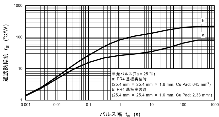
図 9.11 r_{th} - t_w
