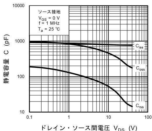
図 9.7 C - V_{DS}
