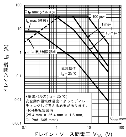
図 9.10 安全動作領域
