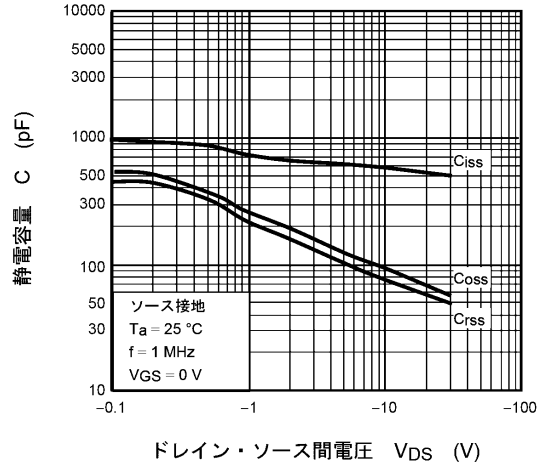
図 9.8 C - V_{DS}
