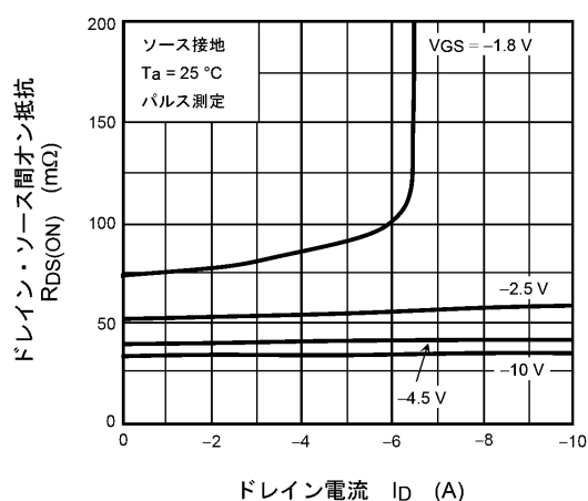
図 9.5 R_{DS(ON)} - I_D
