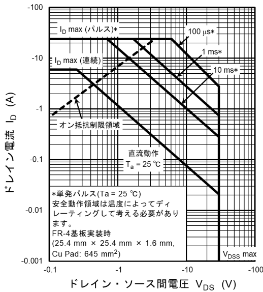
図 9.11 安全動作領域
