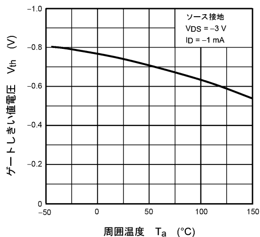
図 9.7 V_{th} - T_a
