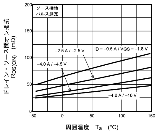
図 9.6 R_{DS(ON)} - T_a
