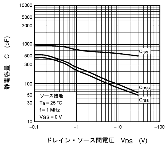
図 9.8 C - V_{DS}
