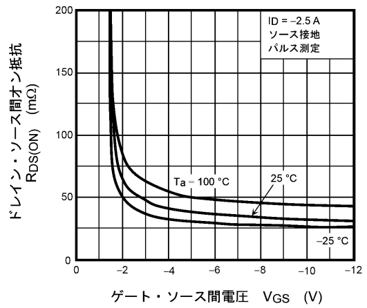
図 9.4 R_{DS(ON)} - V_{GS}
