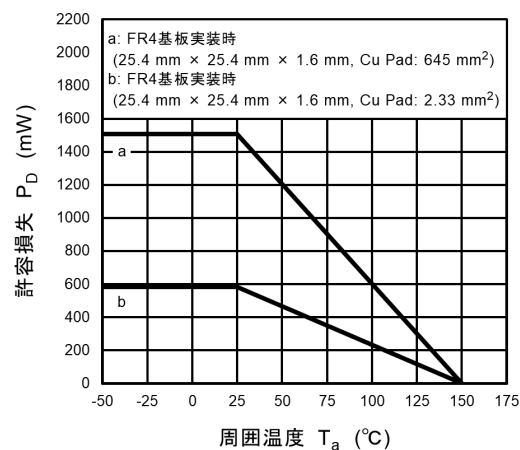
図 9.10 P_D - T_a
