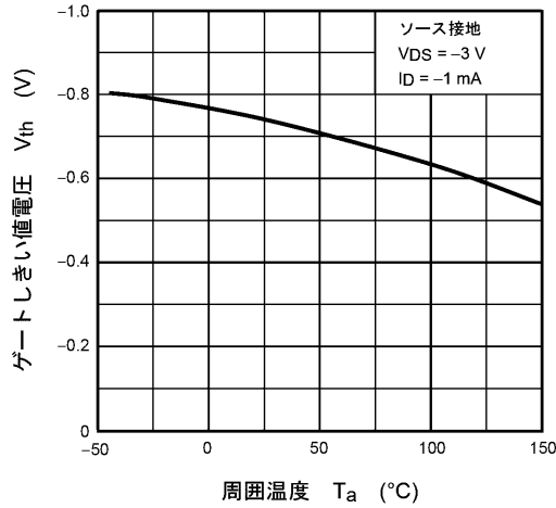
図 9.7 V_{th} - T_a
