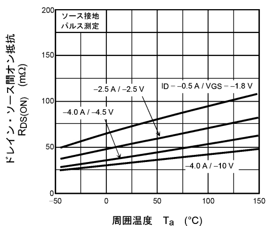
図 9.6 R_{DS(ON)} - T_a
