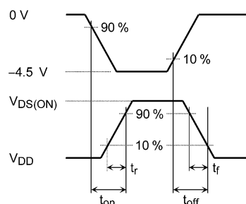
図 6.2.2 入力波形/出力波形
