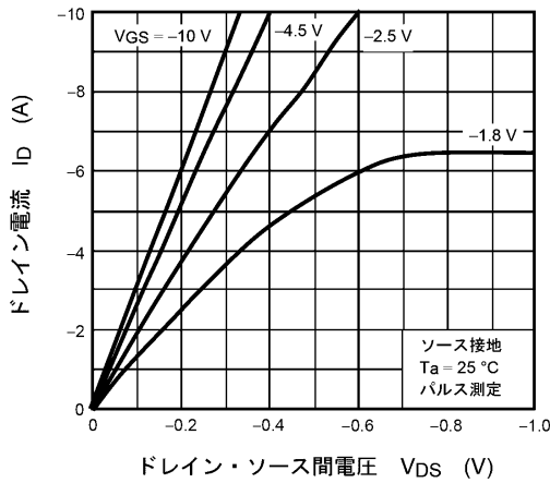
図 9.1 I_D - V_{DS}
