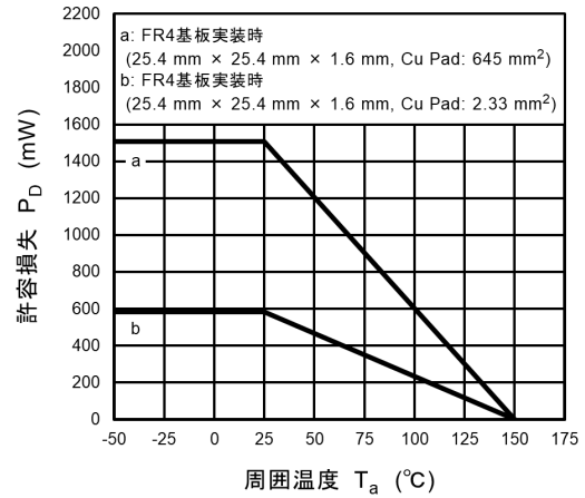
図 9.10 P_D - T_a
