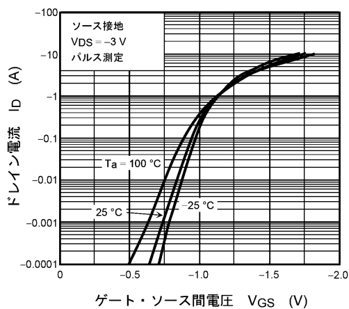
図 9.2 I_D - V_{GS}
