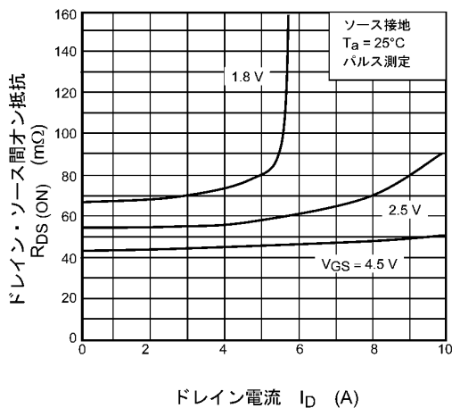
図 9.5 R_{DS(ON)} - I_D
