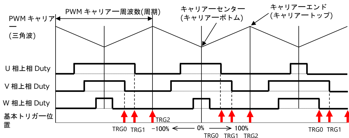
図 10.17 1 シャント、PWM 周期後半、3相変調時のトリガー位置
