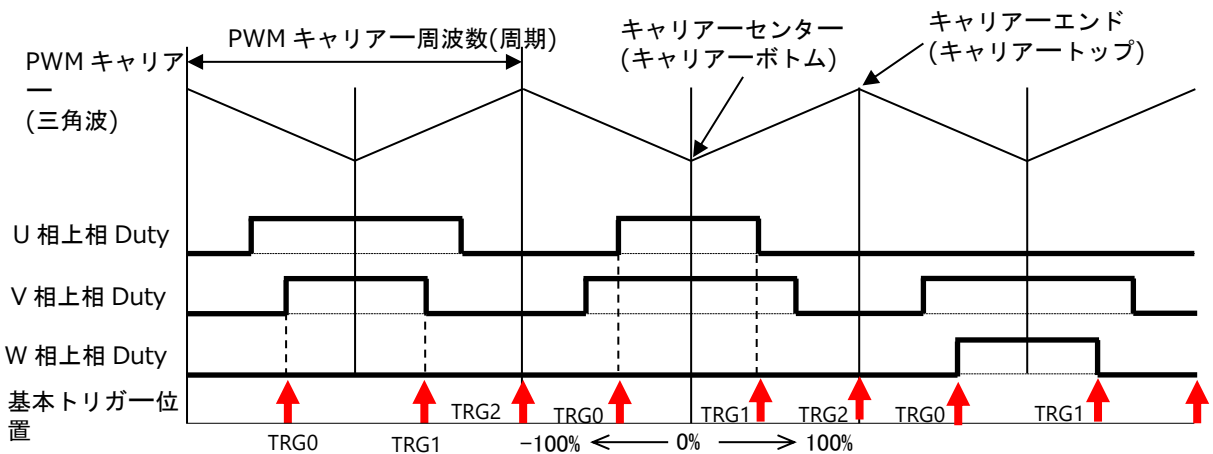
図 10.14 1 シヤント、PWM 周期前半、2 相変調時のトリガー位置
