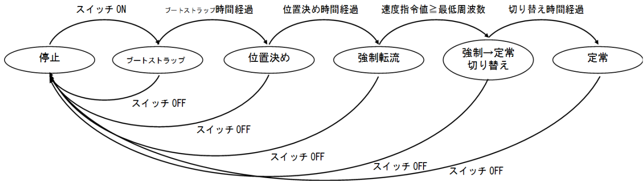
図 10.1 モーター制御の状態遷移図
