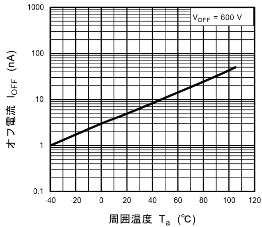
図 12.7 I_{OFF} - T_a
