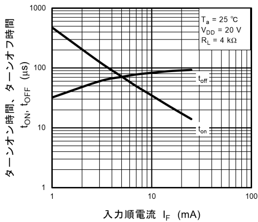
図 12.5 t_{ON}, t_{OFF} - I_F
