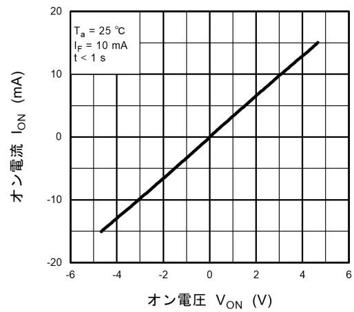
図 12.4 V_{ON} - I_{ON}
