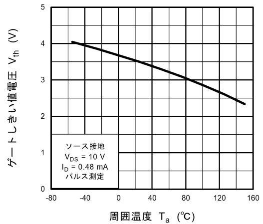
図 8.10 V_{th} - T_a
