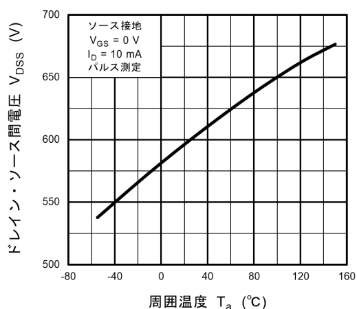
図 8.5 V_{DS} - T_a
