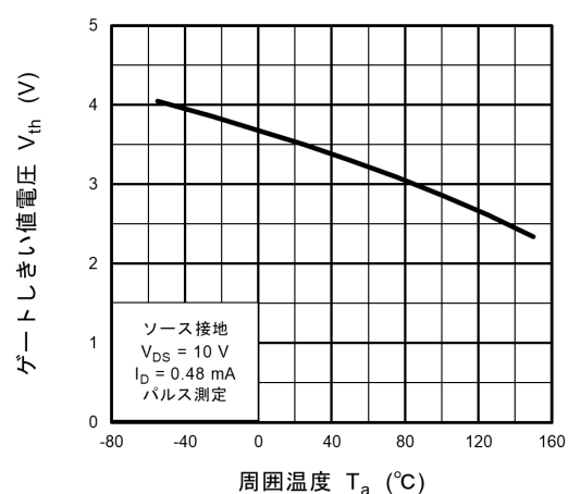
図 8.10 V th - T a
