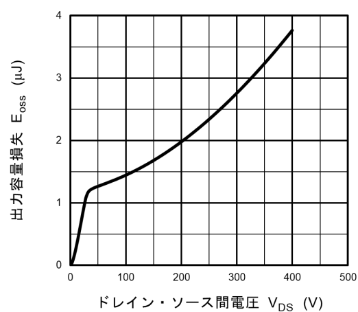
図 8.12 E oss - V DS
