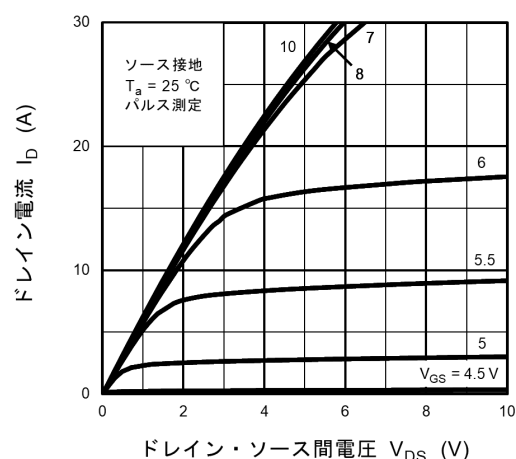
図 8.2 I_D - V_{DS}
