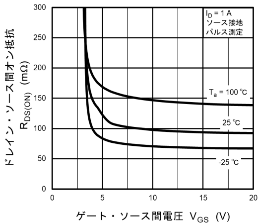
図 9.3 R_{DS(ON)} - V_{GS}
