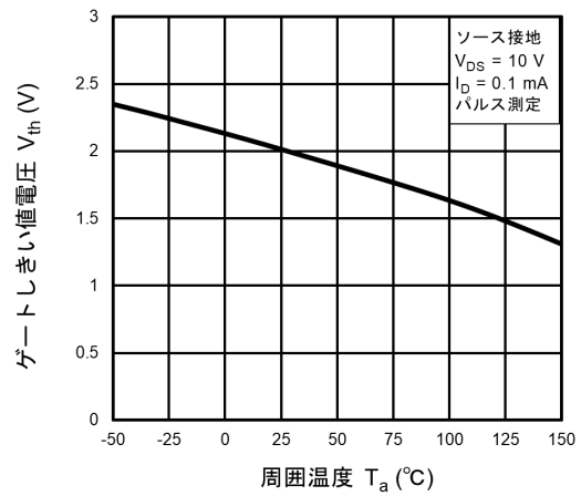
図 9.6 V_{th} - T_a
