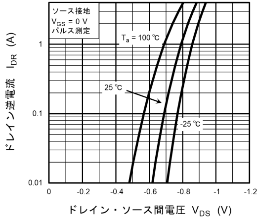
図 9.7 I D - V DS
