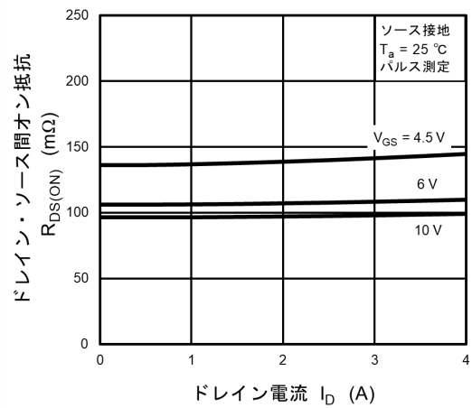
図 9.4 R_{DS(ON)} - I_D
