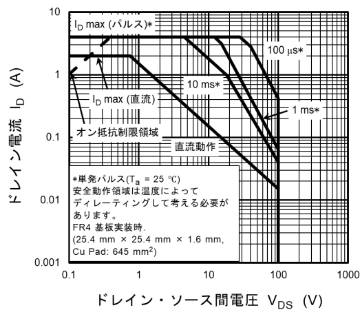
図 9.13 安全動作領域
