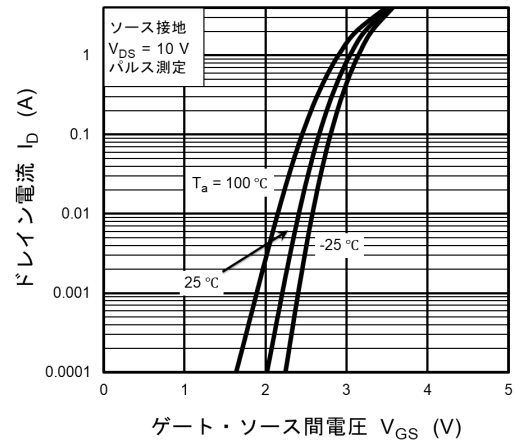
図 9.2 I_D - V_{GS}
