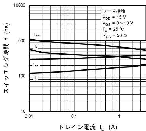
図 9.9 t - I_D
