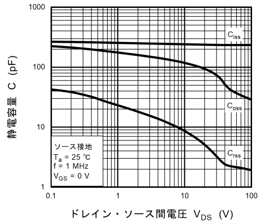
図 9.8 C - V_{DS}
