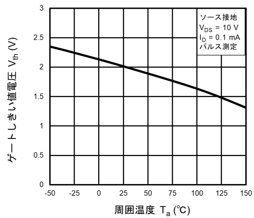
図 9.6 V_{th} - T_a
