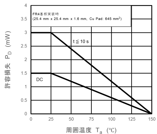
図 9.12 P_D - T_a
