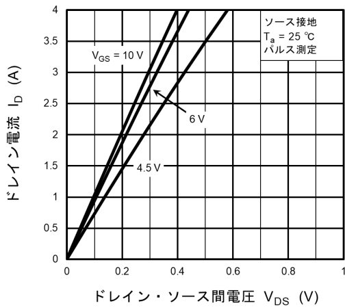
図 9.1 I_D - V_{DS}
