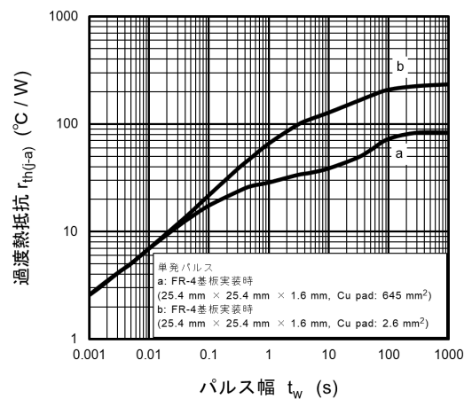
図 9.11 r_{th(j-a)} - t_w
