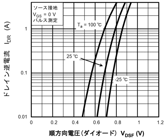
図 9.7 I_{DR} - V_{DSF}
