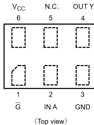
端子配置図
