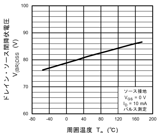
図 8.7 V_{(BR)DSS} - T_a
