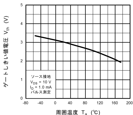
図 8.8 V_{th} - T_a
