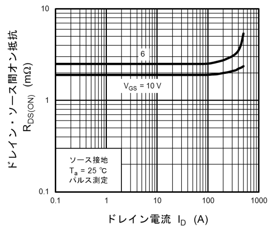
図 8.4 R_{DS(ON)} - I_D
