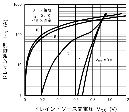
図 8.5 I_{DR} - V_{DS}
