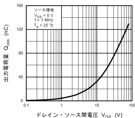
図 8.12 Q_{oss} - V_{DS}
