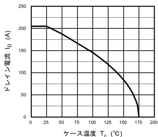
図 8.15 I_D - T_c
