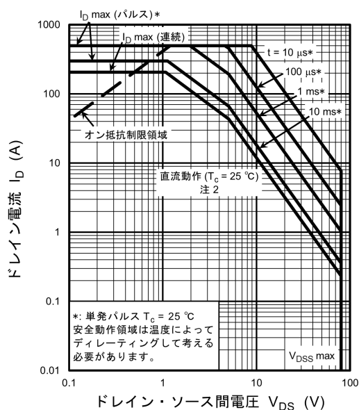
図 8.16 安全動作領域 (最大値 (保証値))
