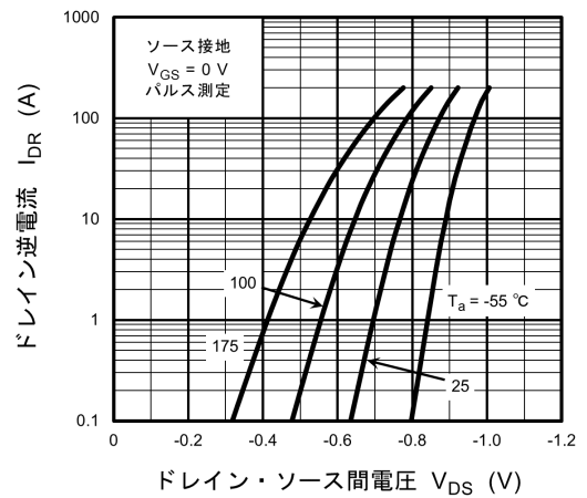
図 8.6 I_{DR} - V_{DS}
