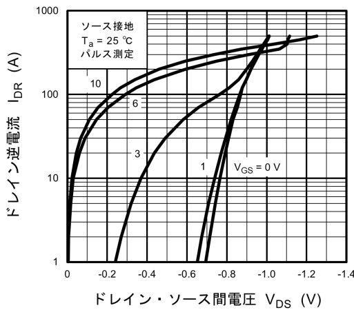
図 8.5 I_{DR} - V_{DS}
