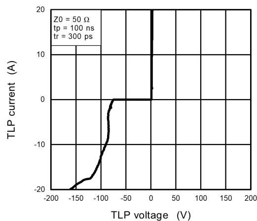
Fig. 10.5.1 I_{TLP} - V_{TLP}
