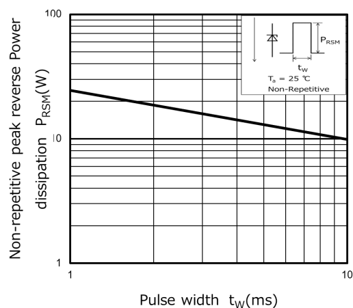
Fig. 10.1.2 P_{RSM} - t_w
