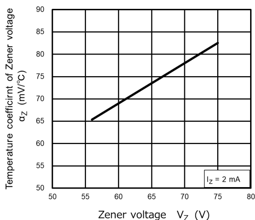
Fig. 10.1.4 \alpha_Z - V_Z
