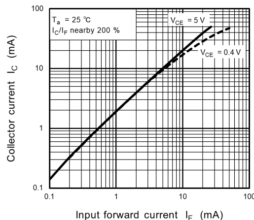
Fig. 12.11 I_C - I_F
