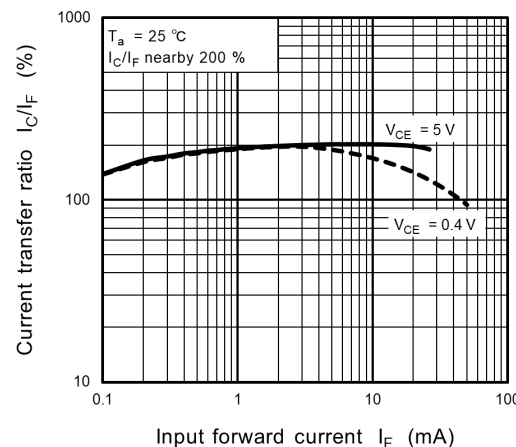
Fig. 12.12 I_C/I_F - I_F
