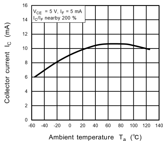
Fig. 12.13 I_C - T_a
