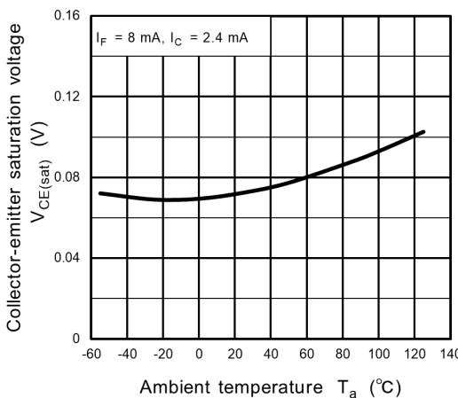
Fig. 12.10 V_{CE(sat)} - T_a
