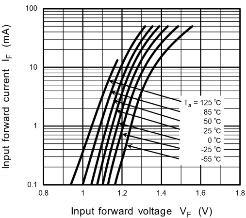
Fig. 12.4 I_F - V_F
