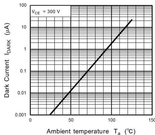
Fig. 12.9 I_{DARK} - T_a
