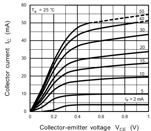
Fig. 12.8 I_C - V_{CE}
