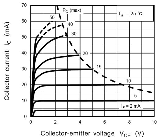
Fig. 12.7 I_C - V_{CE}
