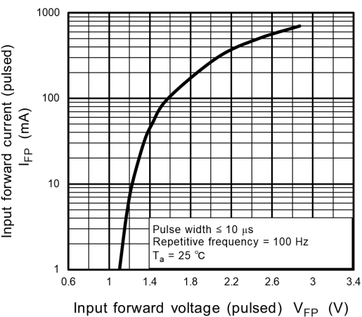
Fig. 12.6 I_{FP} - V_{FP}
