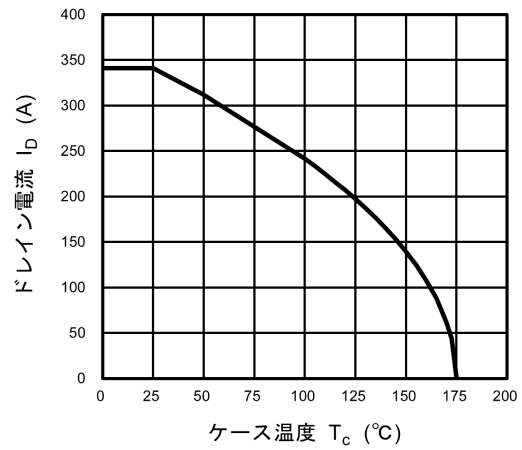
図 8.15 I_D - T_c
