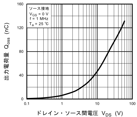
図 8.12 Q_{oss} - V_{DS}
