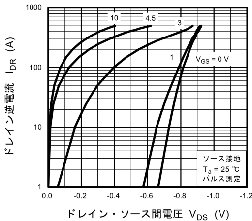
図 8.5 I_{DR} - V_{DS}
