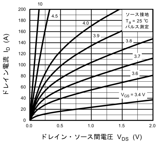
図 8.1 I_D - V_{DS}
