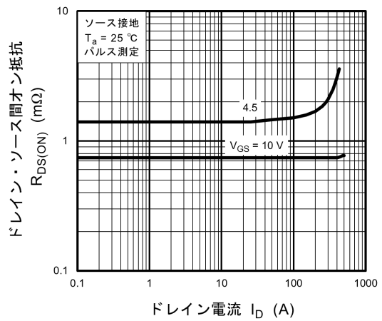
図 8.4 R_{DS(ON)} - I_D
