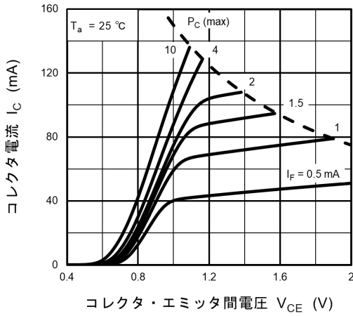
図 12.7 I_C - V_{CE}
