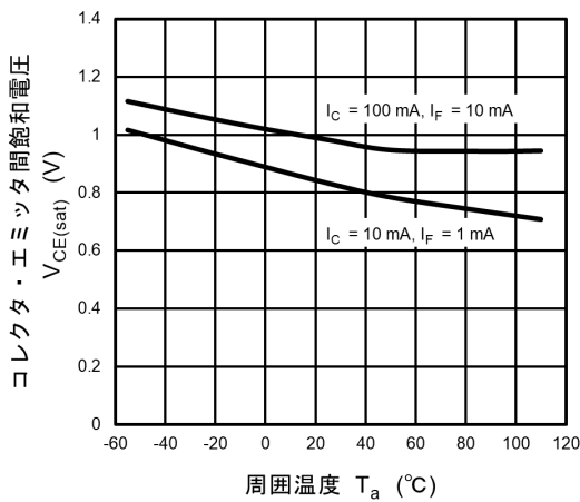
図 12.9 V_{CE(\text{sat})} - T_a
