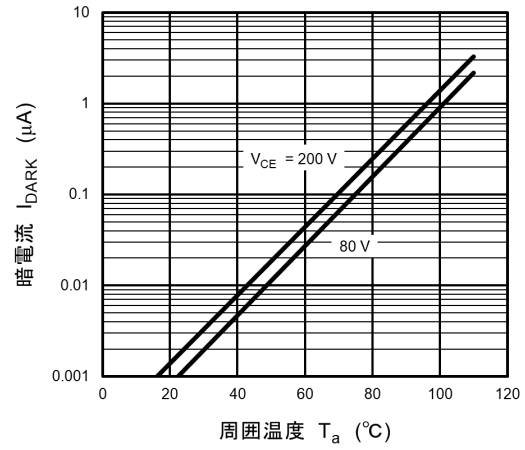
図 12.8 I_{\text{DARK}} - T_a
