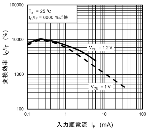
図 12.11 I_C/I_F - I_F
