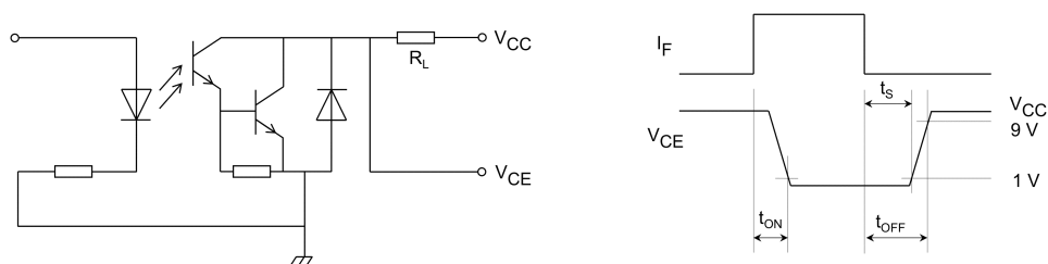
図 11.1 スイッチング時間測定回路, 波形
