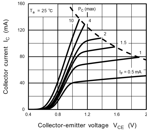
Fig. 12.7 I_C - V_{CE}
