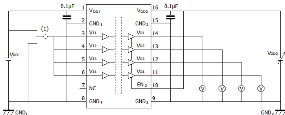
Fig.12.1.7. DCL540L01A/DCL540H01A V_{DD2UV+} / V_{DD2UV-} -Test Circuit
