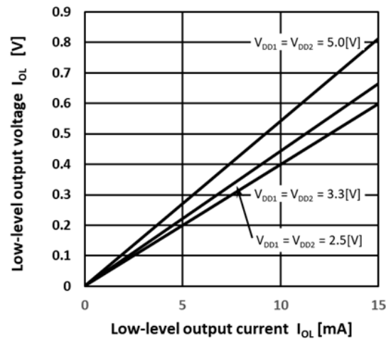
Fig.13.6. V_{OL} - I_{OL}
