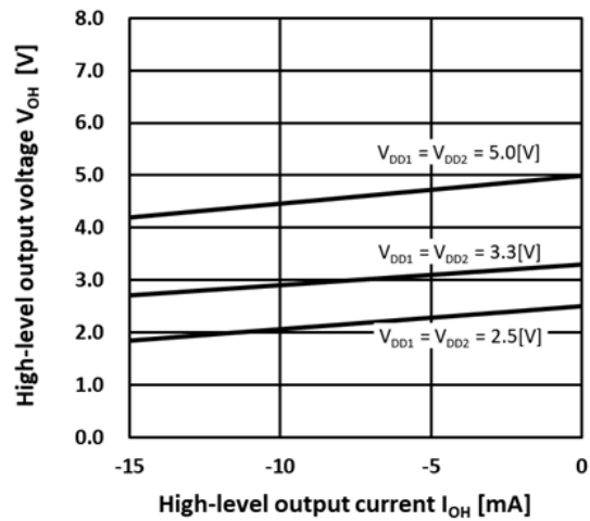
Fig.13.5. V_{OH} - I_{OH}
