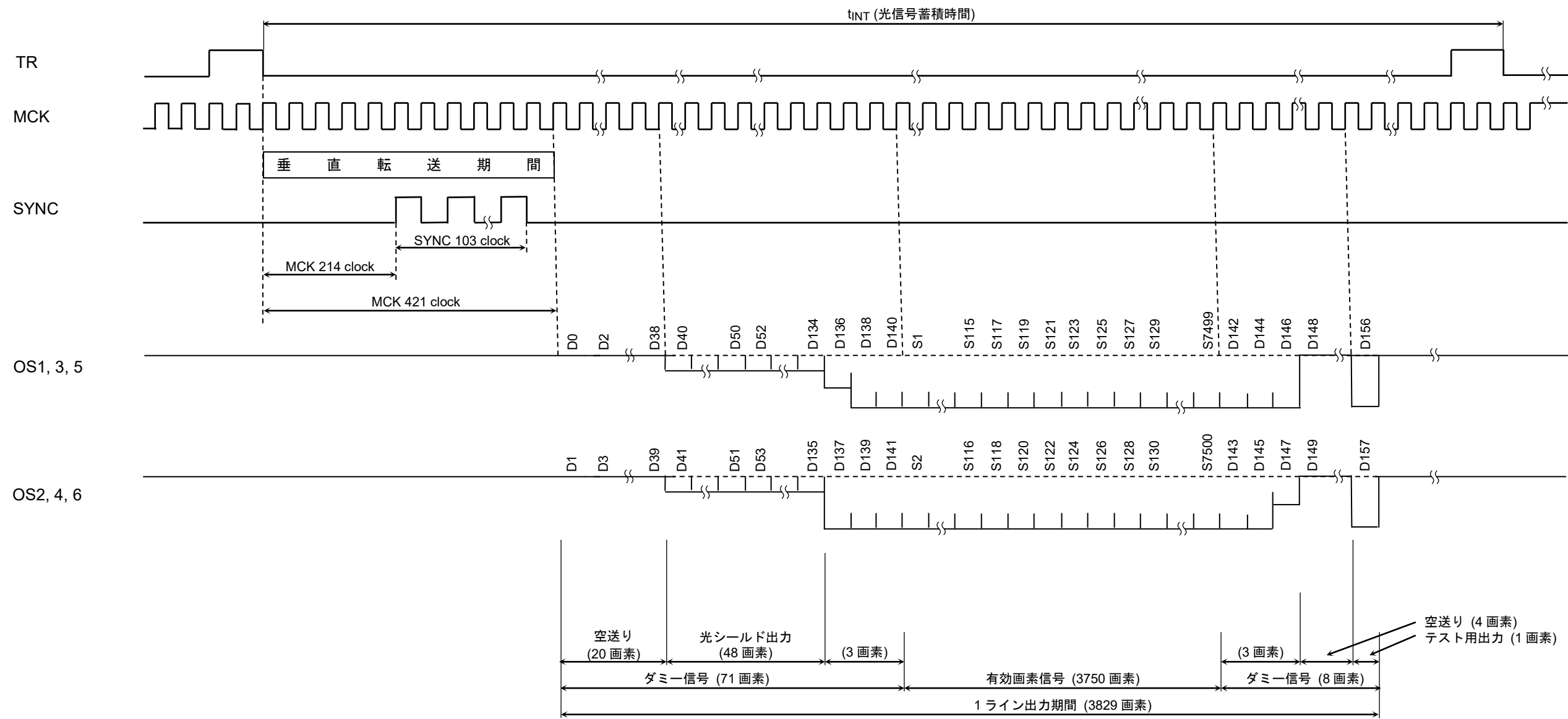
タイミング図:
