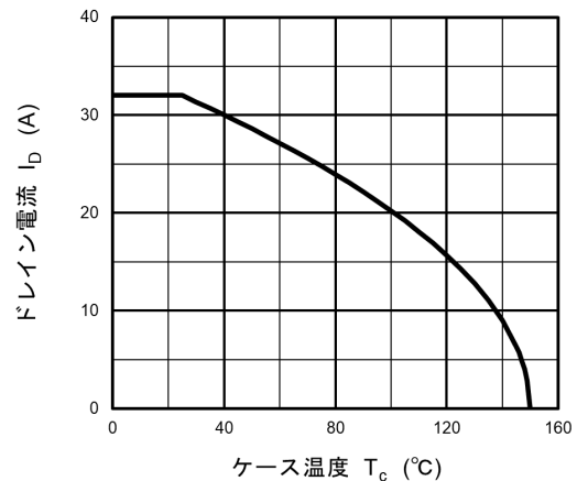
図 8.17 I_D - T_c (最大値 (保証値))
