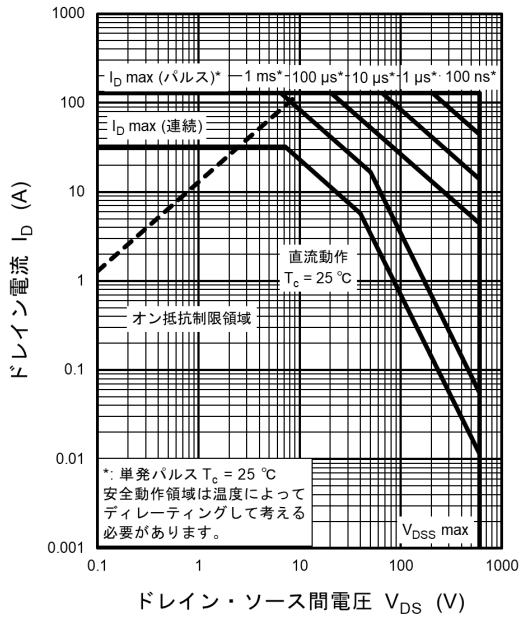
図 8.18 安全動作領域 (最大値 (保証値))
