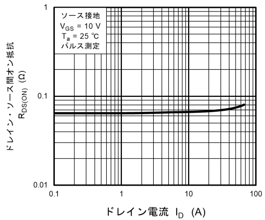
図 8.6 R_{DS(ON)} - I_D
