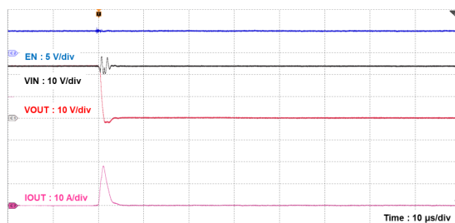
図 12.16 TCKE603RL 短絡保護時の波形 (拡大)
