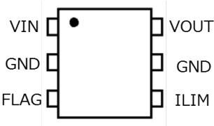
図 3.1 端子配置図 TCKE601RA,TCKE601RL
