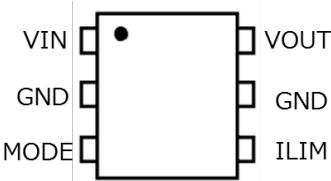
図 3.2 端子配置図 TCKE602RM
