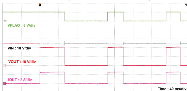
図 12.13 TCKE601RA 短絡保護時の波形 (オートリトライ)
