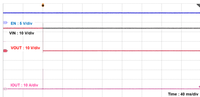
図 12.17 TCKE601RA 過電圧保護時の波形
