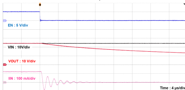
図 12.12 TCKE603RL 過電流保護時の波形 (ラッチ)
