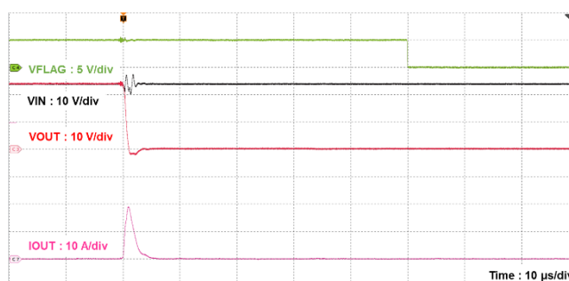
図 12.14 TCKE601RA 短絡保護時の波形 (拡大)
