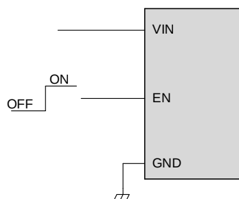
図 9.8.1 EN 端子の接続例 (外部制御)
