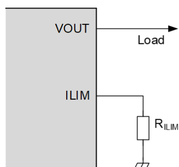
図 9.2.3.1 ILIM 端子周辺外付け回路
