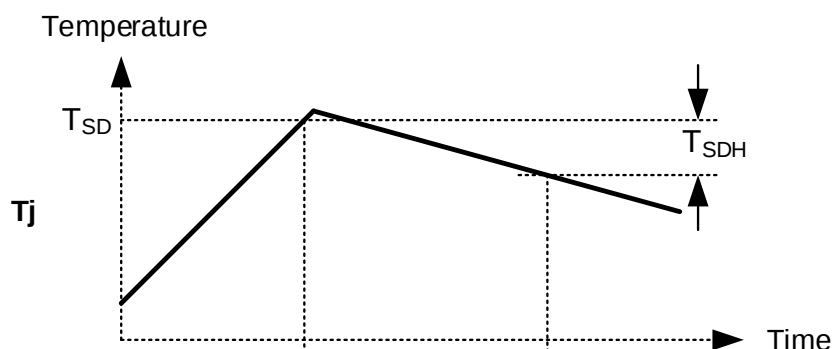
図 9.5.1 過熱保護動作
