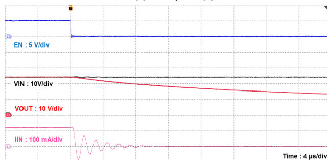
図 12.10 出力立ち下がり波形 V_{IN} = 24\text{ V} , C_{OUT} = 1\text{ }\mu\text{F} , R_{OUT} = 200\text{ }\Omega
