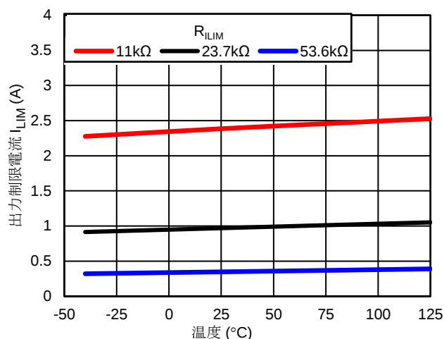
図 12.8 出力制限電流 I_{LIM} V_{IN} = 24\text{ V} , V_{EN} = 3\text{ V}
