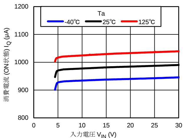
図 12.3 消費電流 (ON 状態) I_Q
