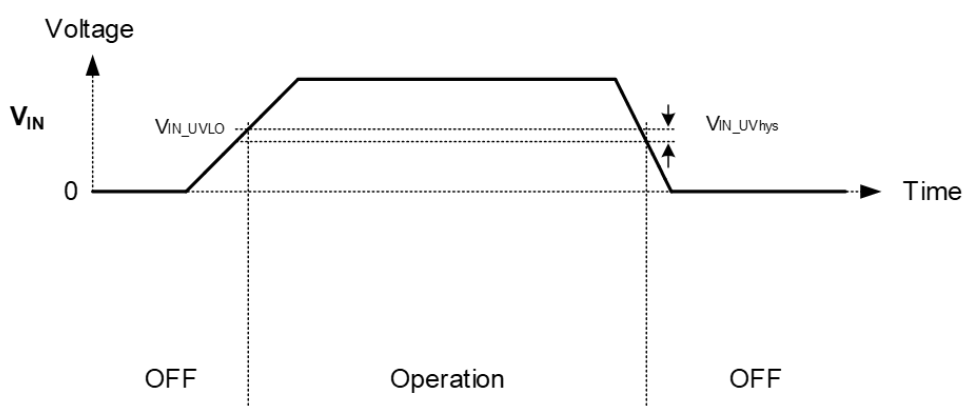
図 9.7.1 波形図
