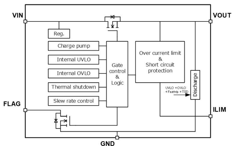
図 7.1 ブロック図 TCKE601RA, TCKE601RL
