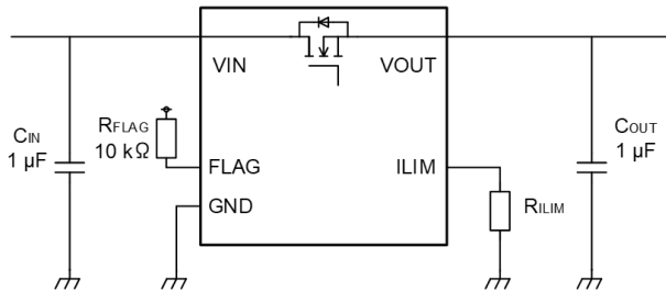
図 10.1.1 TCKE601 の周辺回路例
