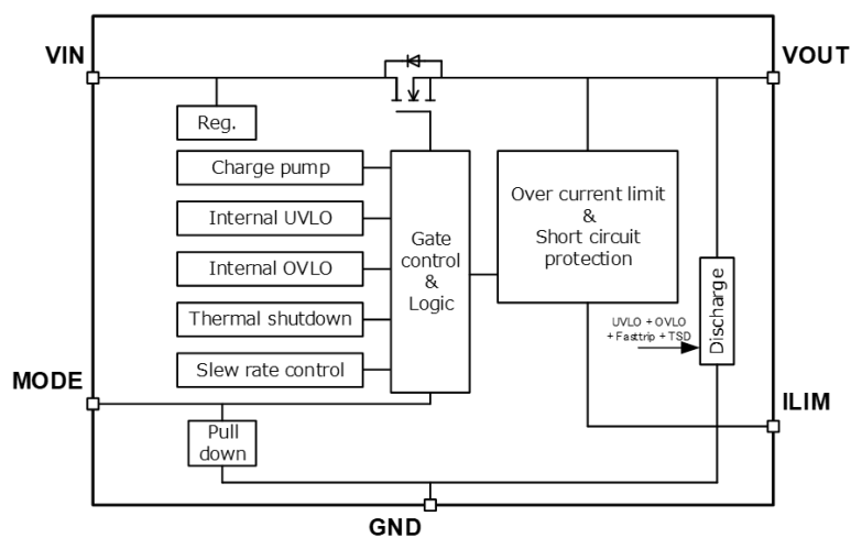
図 7.2 ブロック図 TCKE602RM
