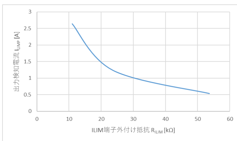
図 9.2.3.2 出力検知電流 I_{LIMP} と ILIM 端子外付け抵抗 R_{ILIM} の関係
