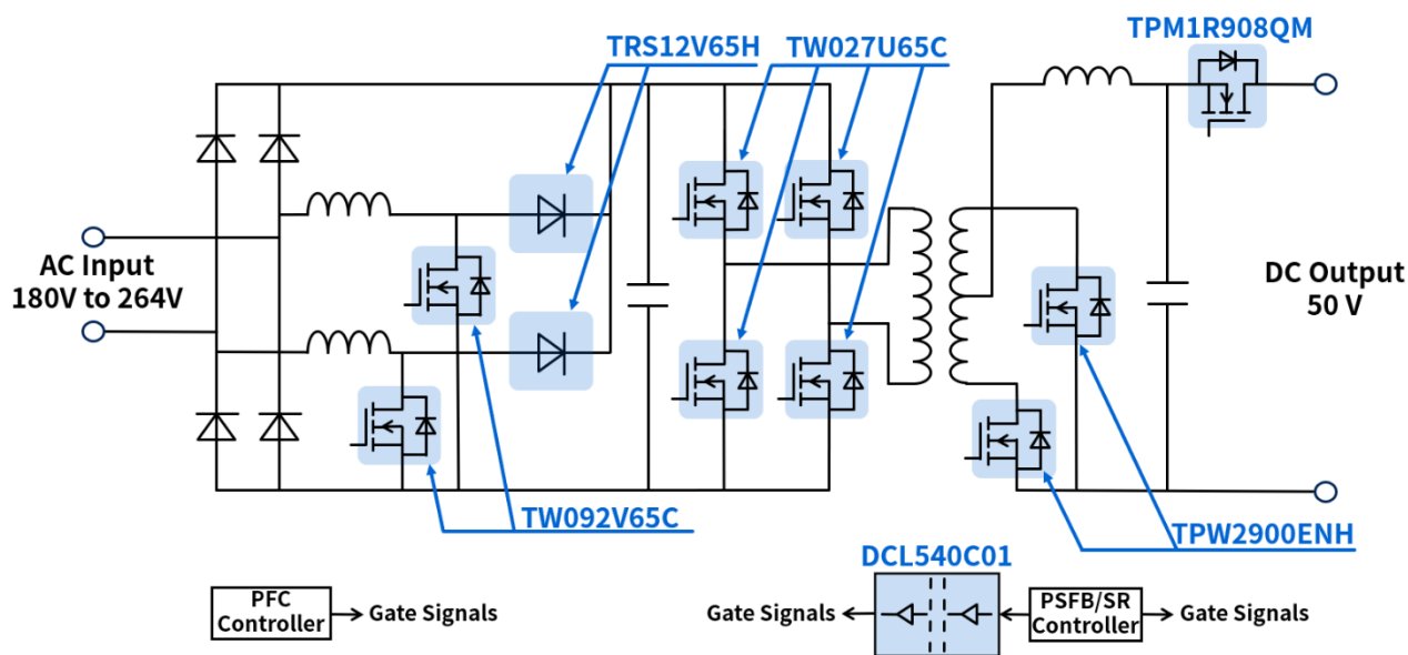
図 2.1 ブロック図
