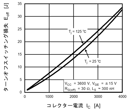
図 7.6 E_{off} - I_C
