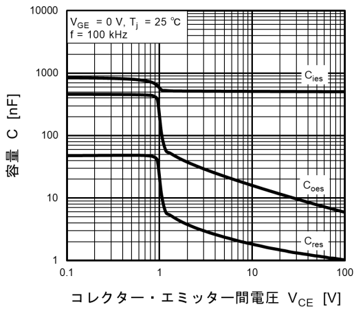
図 7.3 容量 - V_{CE}
