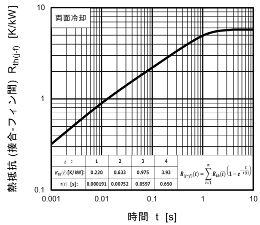
図 7.10 R_{th(j-f)} - t (保障値)
