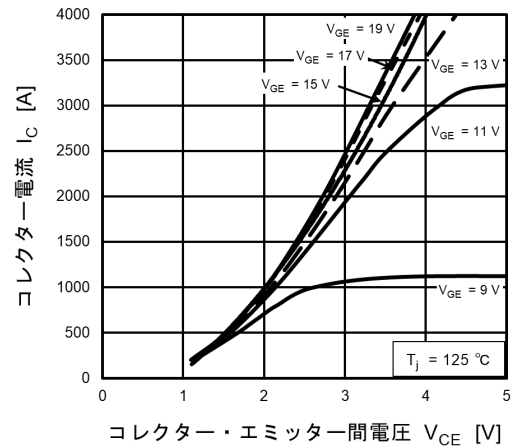
図 7.2 I_C - V_{CE}
