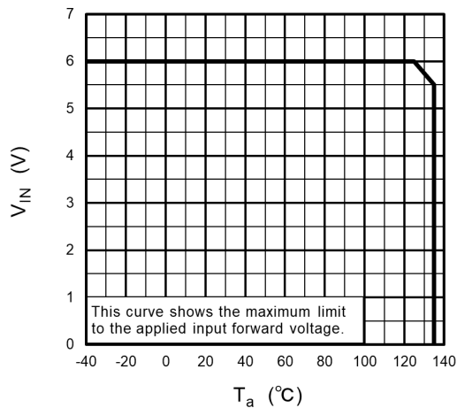
Fig. 12.1 V_{IN} - T_a
