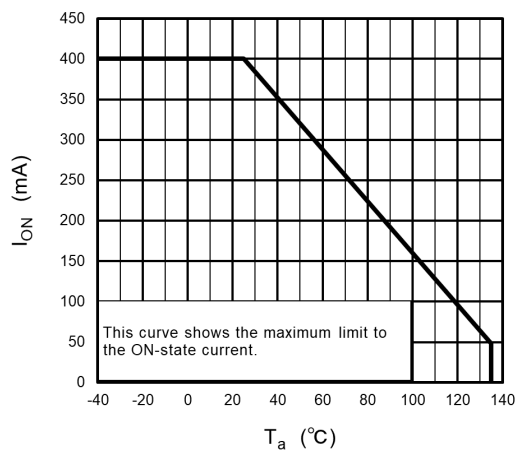
Fig. 12.3 I_{ON} - T_a
