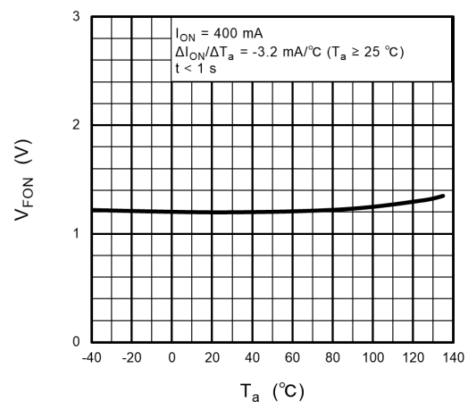
Fig. 12.6 V_{FON} - T_a
