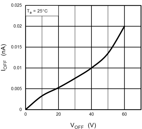
Fig. 12.10 I_{OFF} - V_{OFF}
