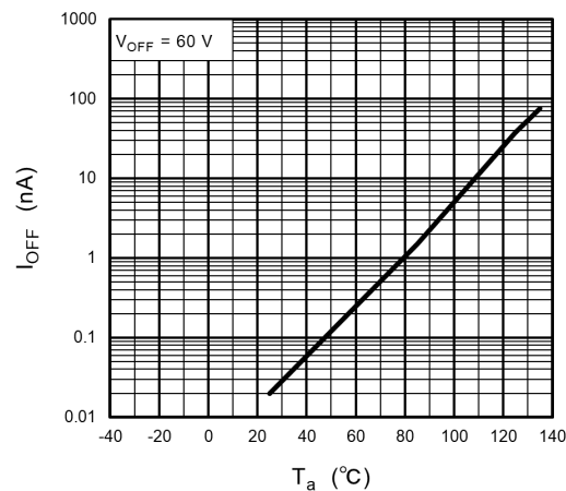
Fig. 12.11 I_{OFF} - T_a
