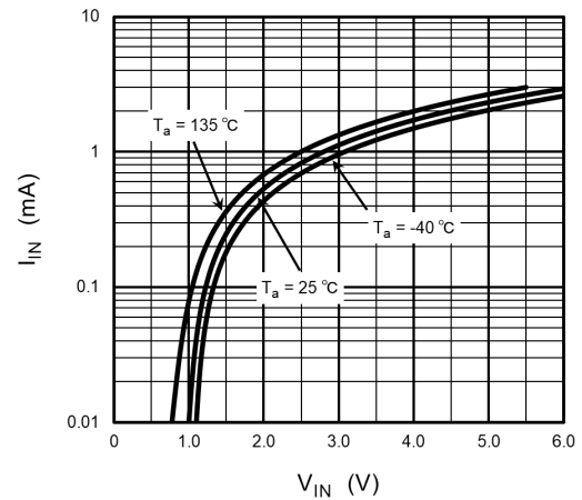
Fig. 12.2 I_{IN} - V_{IN}
