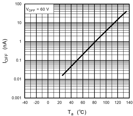
Fig. 12.11 I_{OFF} - T_a
