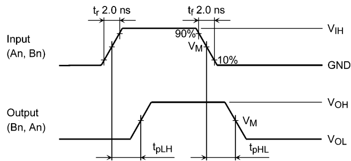
図 13.1 t PLH , t PHL
