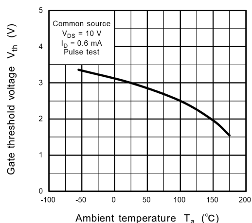
Fig. 8.12 V_{th} - T_a
