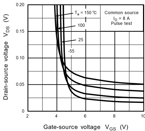
Fig. 8.5 V_{DS} - V_{GS}
