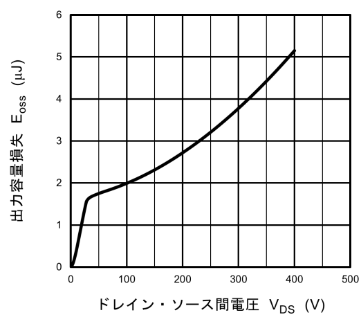
図 8.12 E_{oss} - V_{DS}
