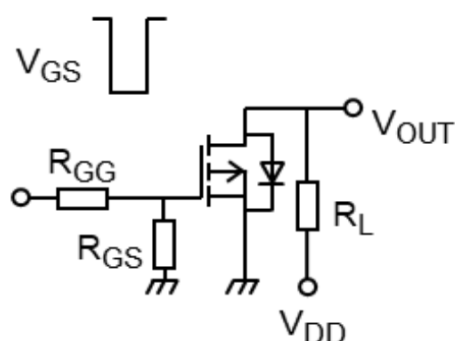
図 6.3.1 スwitchング時間の測定回路
