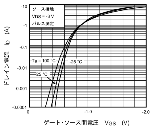
図 8.2 I_D - V_{GS}
