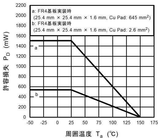
図 8.11 P_D - T_a
