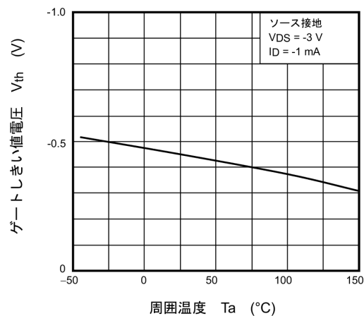
図 8.6 V_{th} - T_a
