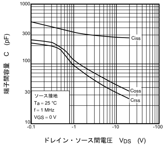
図 8.7 C - V_{DS}
