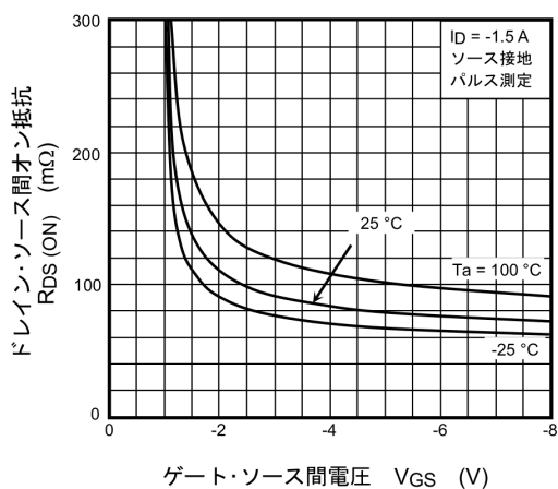
図 8.3 R_{DS(ON)} - V_{GS}
