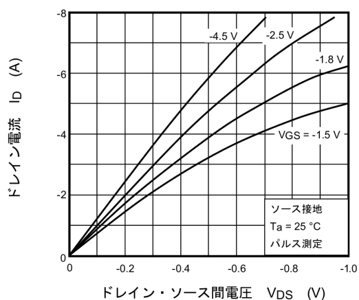
図 8.1 I_D - V_{DS}
