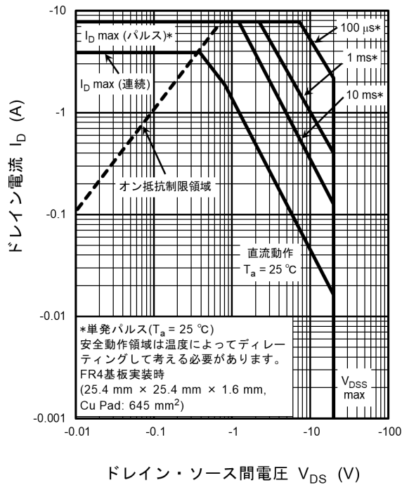
図 8.9 安全動作領域
