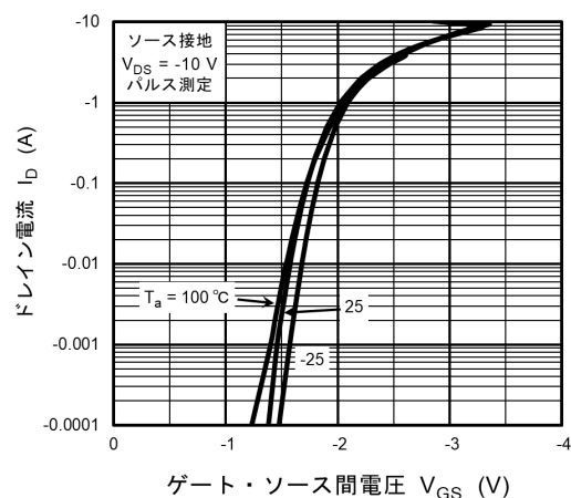
図 8.2 I_D - V_{GS}
