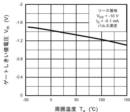
図 8.6 V_{th} - T_a
