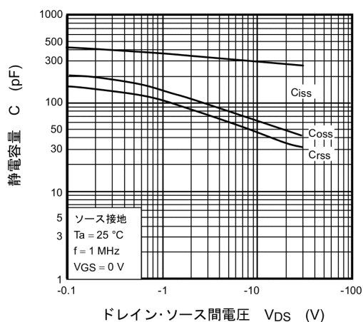
図 8.7 C - V_{DS}
