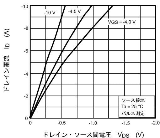
図 8.1 I_D - V_{DS}
