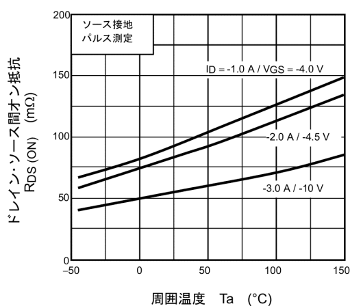
図 8.5 R_{DS(ON)} - T_a
