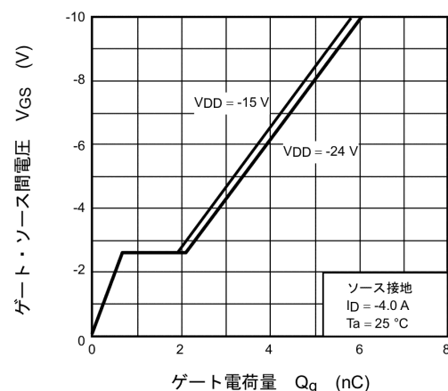
図 8.8 ダイナミック入力特性
