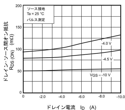
図 8.4 R_{DS(ON)} - I_D
