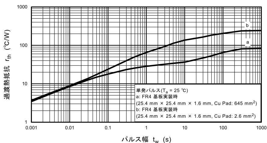
図 8.9 r_{th} - t_w
