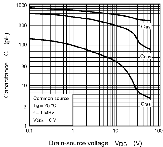
Fig. 8.7 C - V_{DS}
