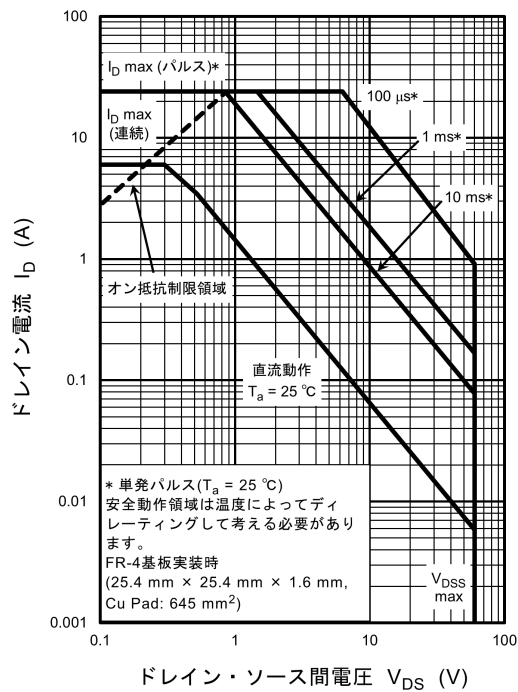
図 8.9 安全動作領域図
