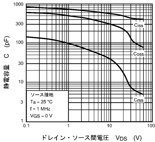
図 8.7 C - V_{DS}
