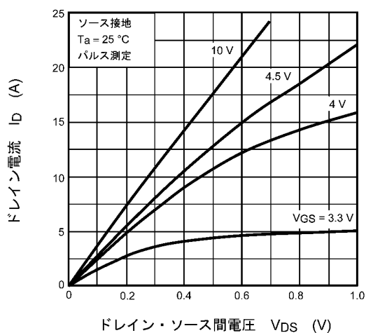
図 8.1 I_D - V_{DS}
