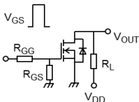
図 6.3.1 スwitchング時間の測定回路
