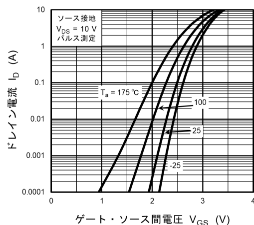
図 8.2 I_D - V_{GS}
