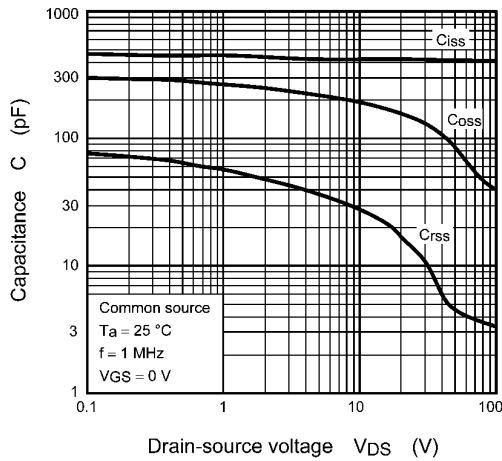
Fig. 8.7 C - V_{DS}
