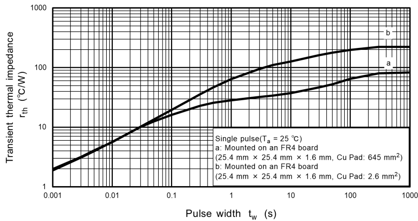
Fig. 8.9 r_{th} - t_w
