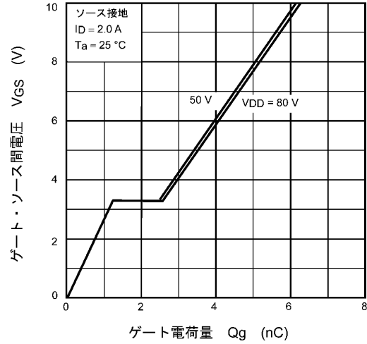
図 8.8 ダイナミック入力特性
