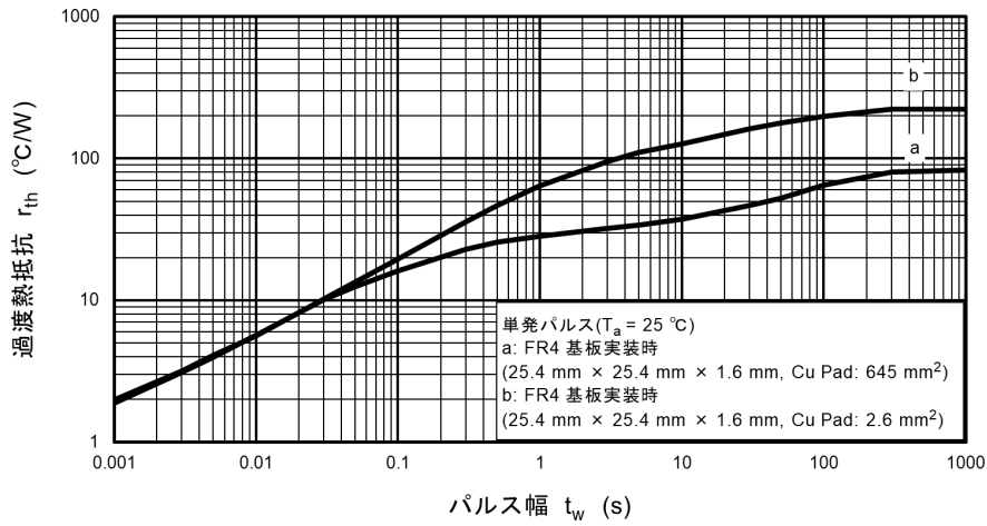
図 8.9 r_{th} - t_w
