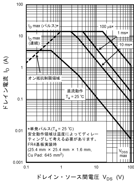
図 8.10 安全動作領域
