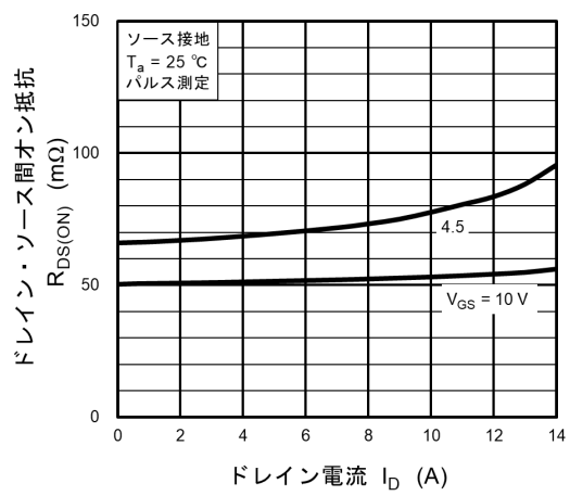
図 8.4 R_{DS(ON)} - I_D
