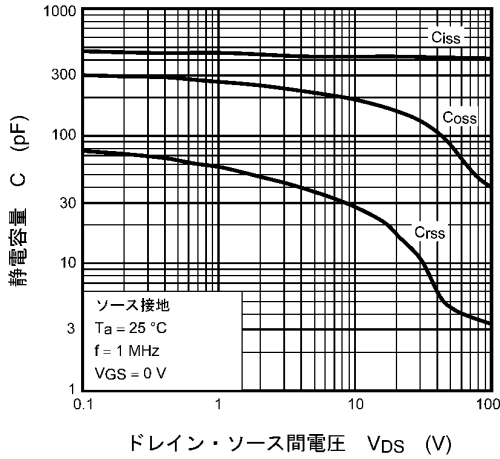
図 8.7 C - V_{DS}
