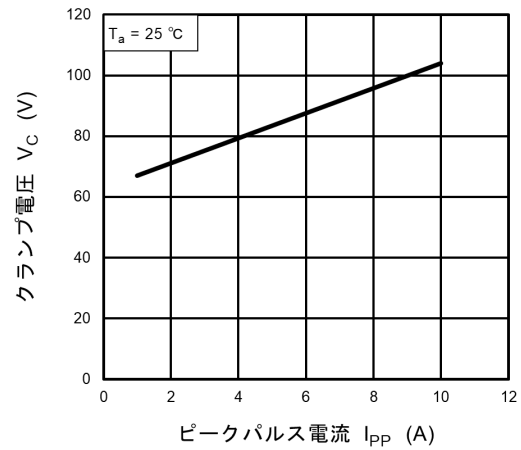
図 10.3.2 V_C - I_{PP}
