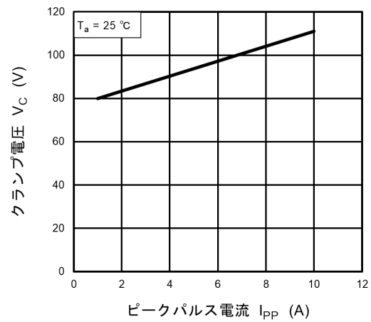
図 10.5.2 V_C - I_{PP}
