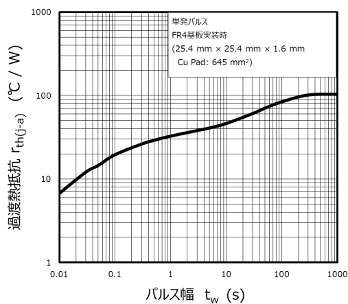
図 10.1.5 r_{th(j-a)} - t_w
