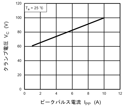
図 10.2.2 V_C - I_{PP}
