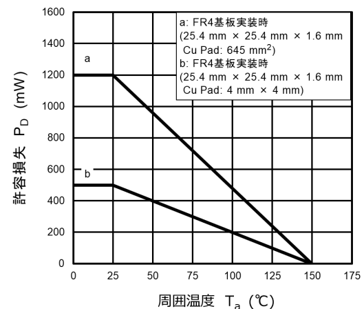
図 10.1.6 P_D - T_a
