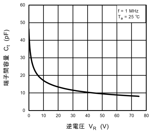
図 10.5.3 C_T - V_R
