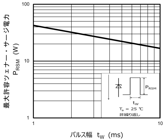
図 10.1.2 P_{RSM} - t_w
