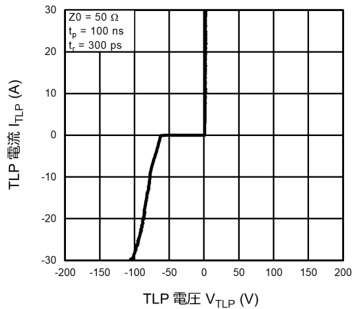
図 10.3.1 I_{TLP} - V_{TLP}
